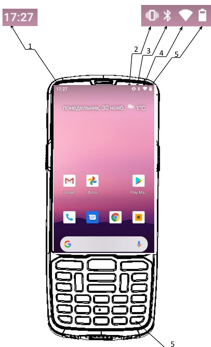
Рисунок 9. Расположение основных индикаторов изделия
